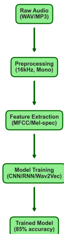
Slika 3: Dijagram toka prikazuje kompletan pipeline od sirovog audio signala do trenirane neuronske mreže
